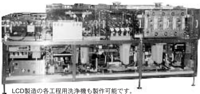
←ブラシ調整部 Brush adjusting part
