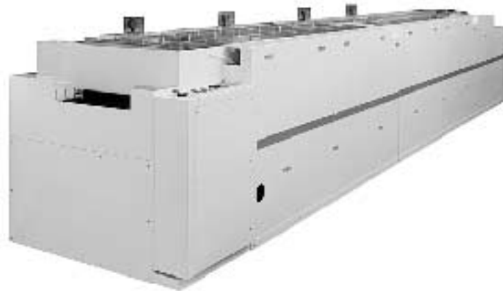
←ブラシ調整部 Brush adjusting part
